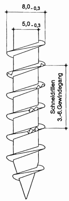
Ansicht Z
