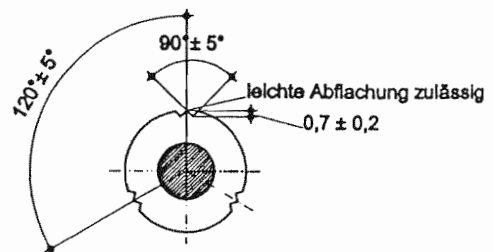
Schnitt
