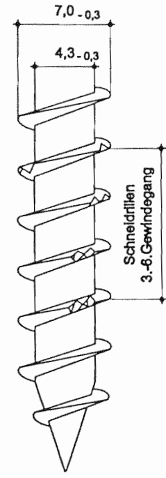
Ansicht Z
