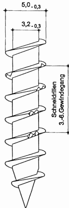
Ansicht Z
