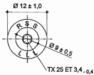
Ansicht X
