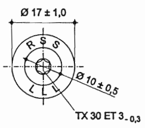
Ansicht X
